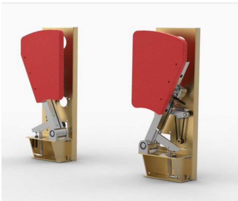
图 1 机芯结构
